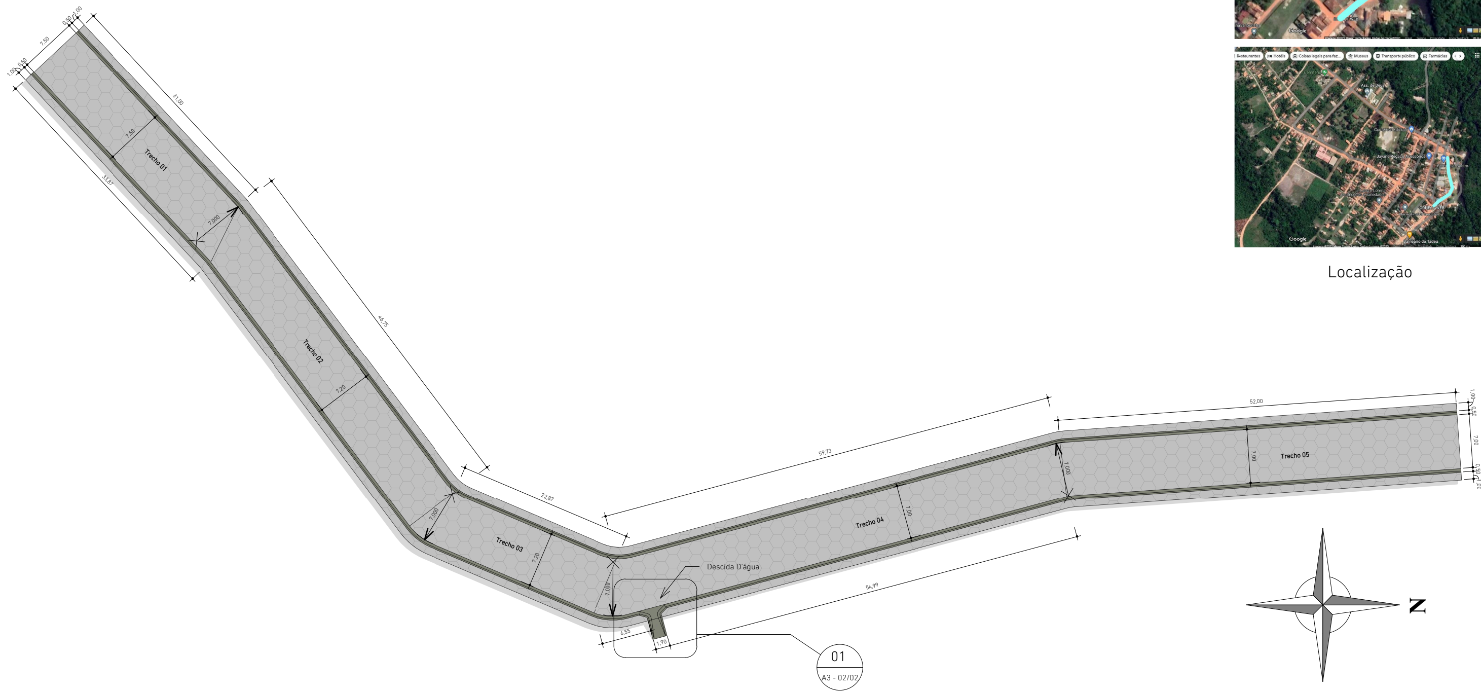
Via Pavimentada - 1 : 500
