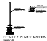
DETALHE 1: PILAR DE MADEIRA Escala 1/50
