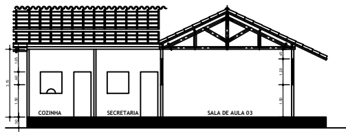
CORTE B-B'
