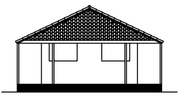
FACHADA FRONTAL
